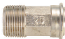
Tubete Curto 3/4 (DN 20) 1 (DN 25)
